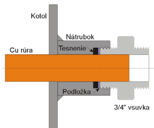
Schéma utesnenia Cu rúry vsuvkou na teleso kotla
