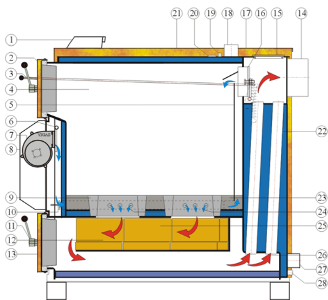
Schéma VIGAS 80
