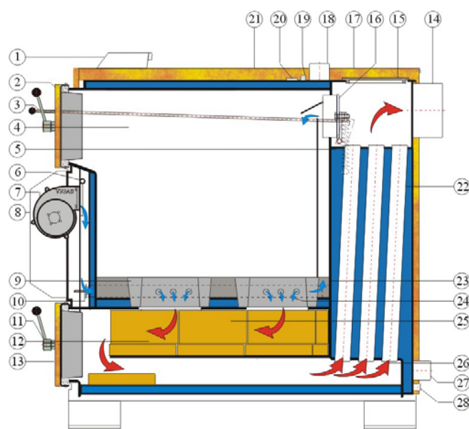
Schéma VIGAS 100
